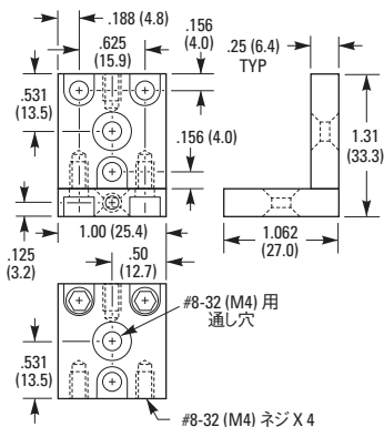
MT-RS 小型回転ステージ
